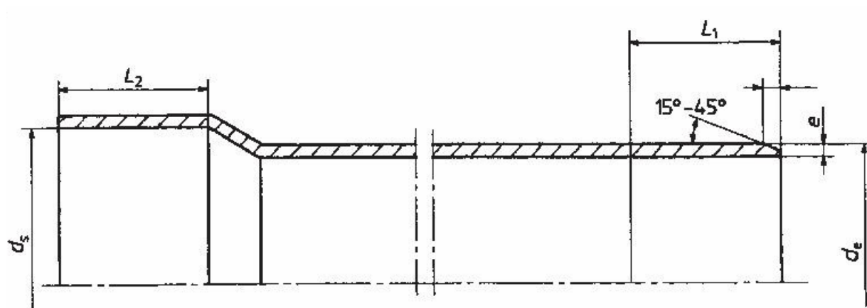
Fig. 2 – Dimensiones básicas de embocaduras para unión por encolado
