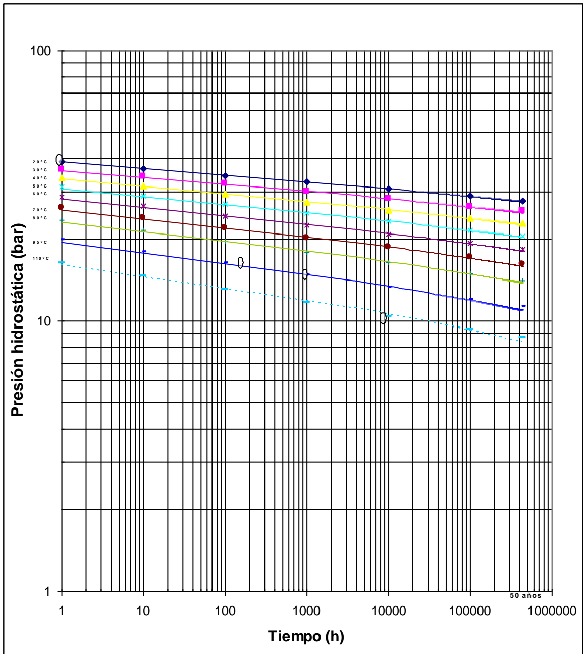
Figura 2 - Líneas de regresión mínima de los tubos multicapa de Polímero Plástico/Al/PE-X
